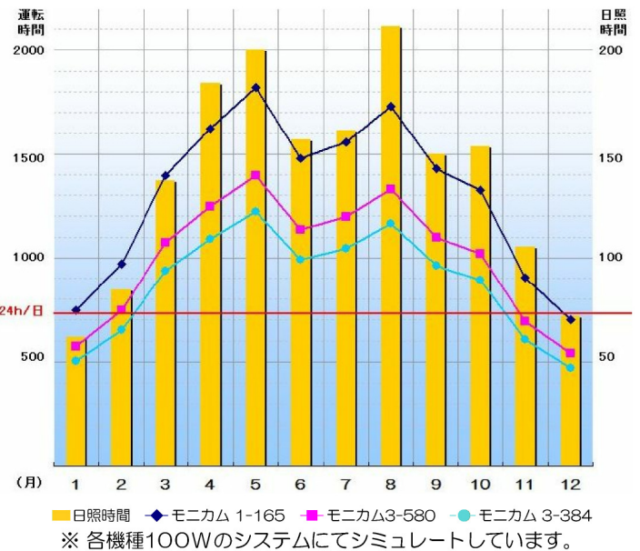
【金沢市の月別平均日照時間と各機種の運転可能時間】
